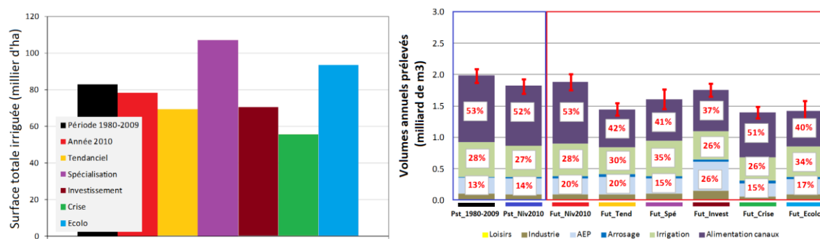
Figure 5 : Evolution de la surface totale irriguée considérée dans MODIC (à gauche) et prélèvements par usage avec MODIC_CF (à droite) selon les six scénarios socio-économiques sous les climats temps présent (Pst) et 2050 (Fut) issus de la sélection de dix projections climatiques régionalisées, à l'échelle du système Durance-Verdon. Les segments en rouge représentent la dispersion induite par les dix climats modélisés
